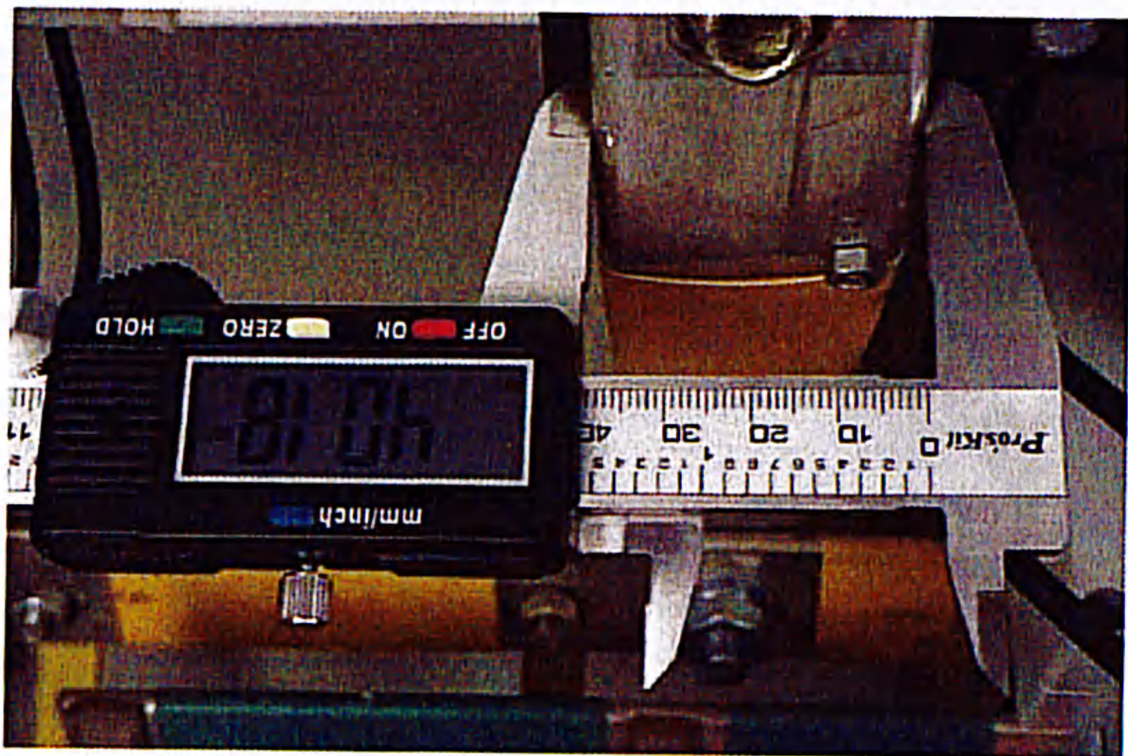
主开关出线排宽度
