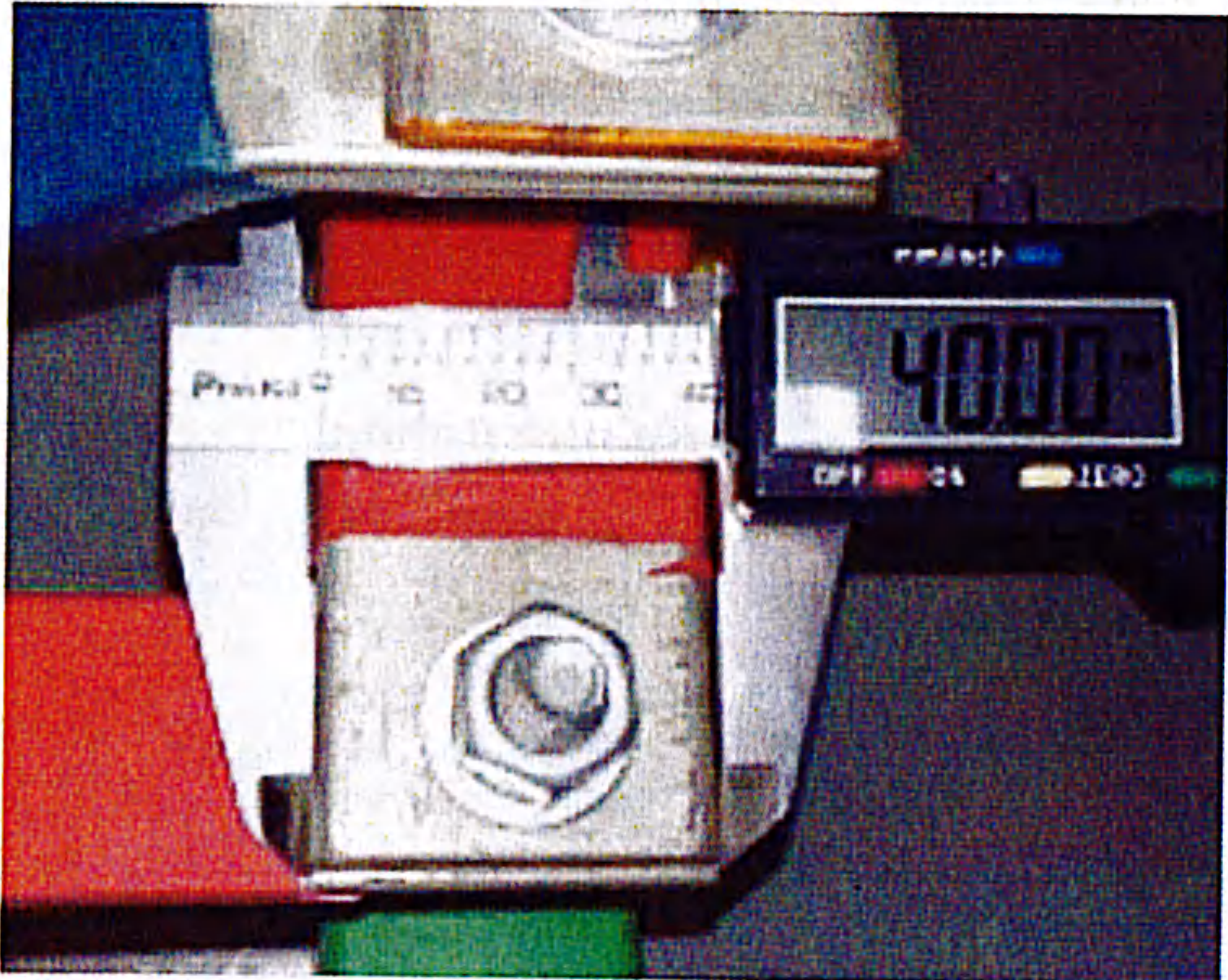
主母线宽度
